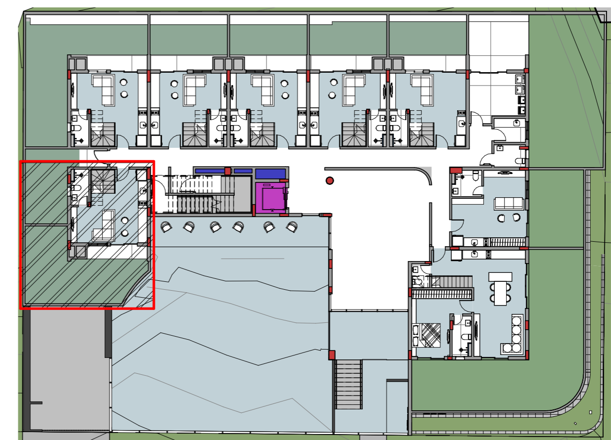
1 - E-01 - TÉRREO - 111 ESCALA 1 : 250
