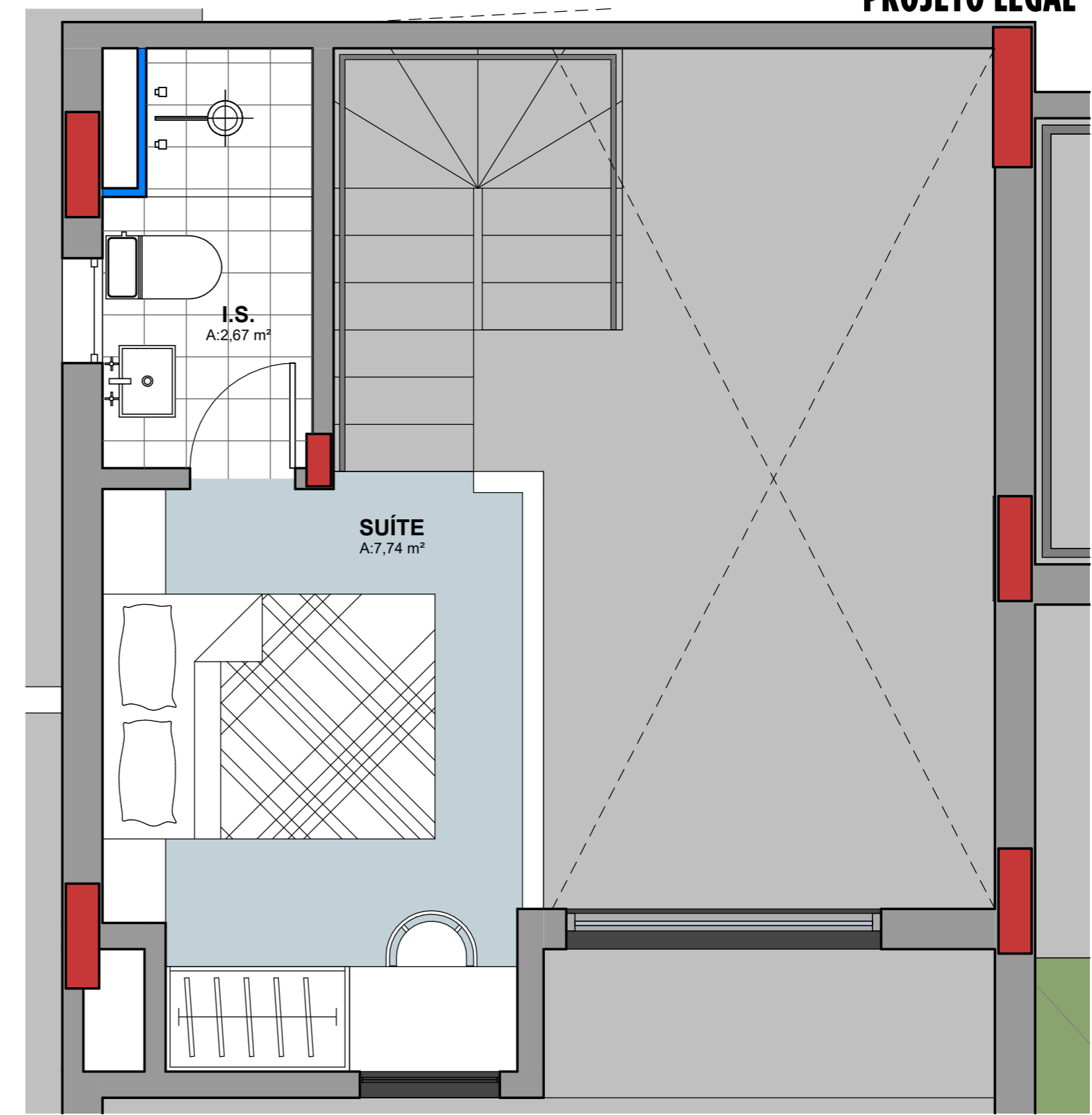
MEZANINO - APTO 111 ESCALA 1 : 30
