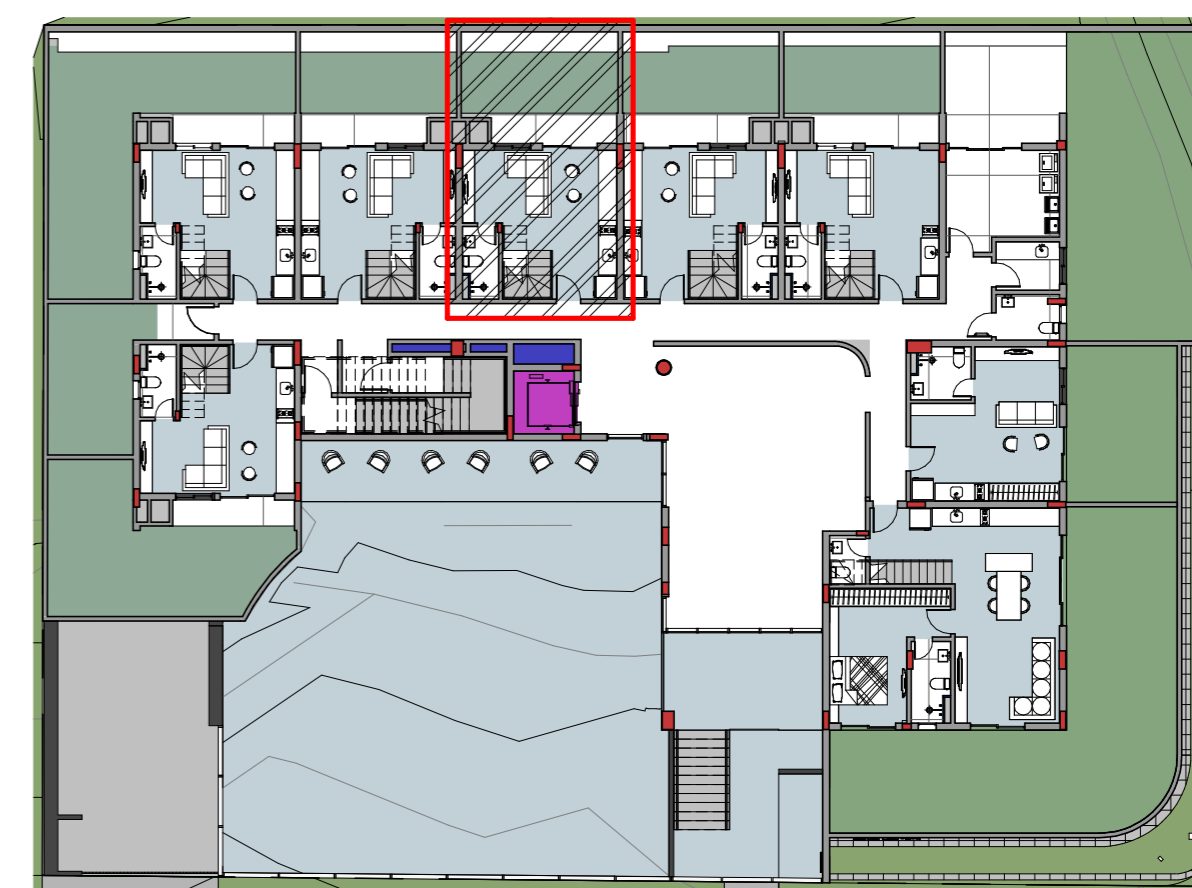
1 - E-01 - TÉRREO - 108 ESCALA 1 : 250
