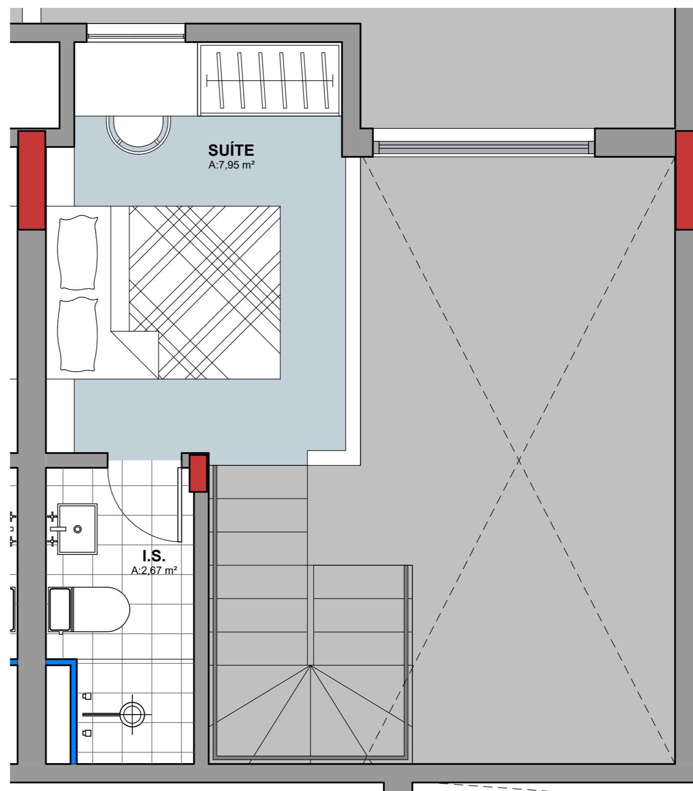
MEZANINO - APTO 108 ESCALA 1 : 30
