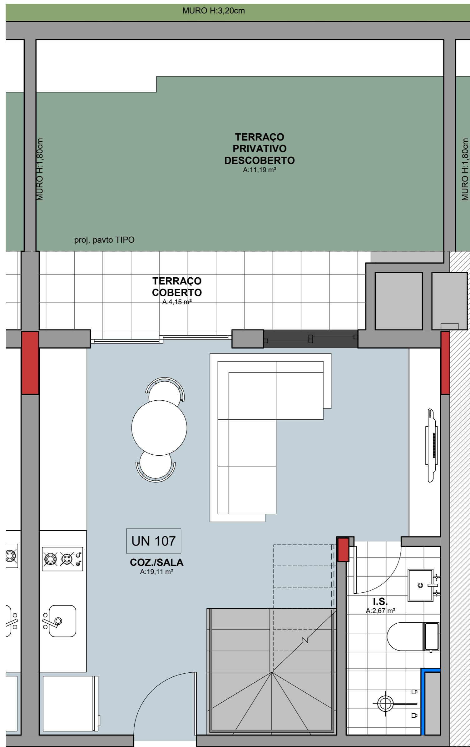
APTO 107 ESCALA 1 : 30
