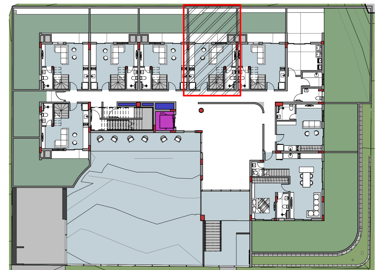
1 - E-01 - TÉRREO - 107 ESCALA 1 : 250
