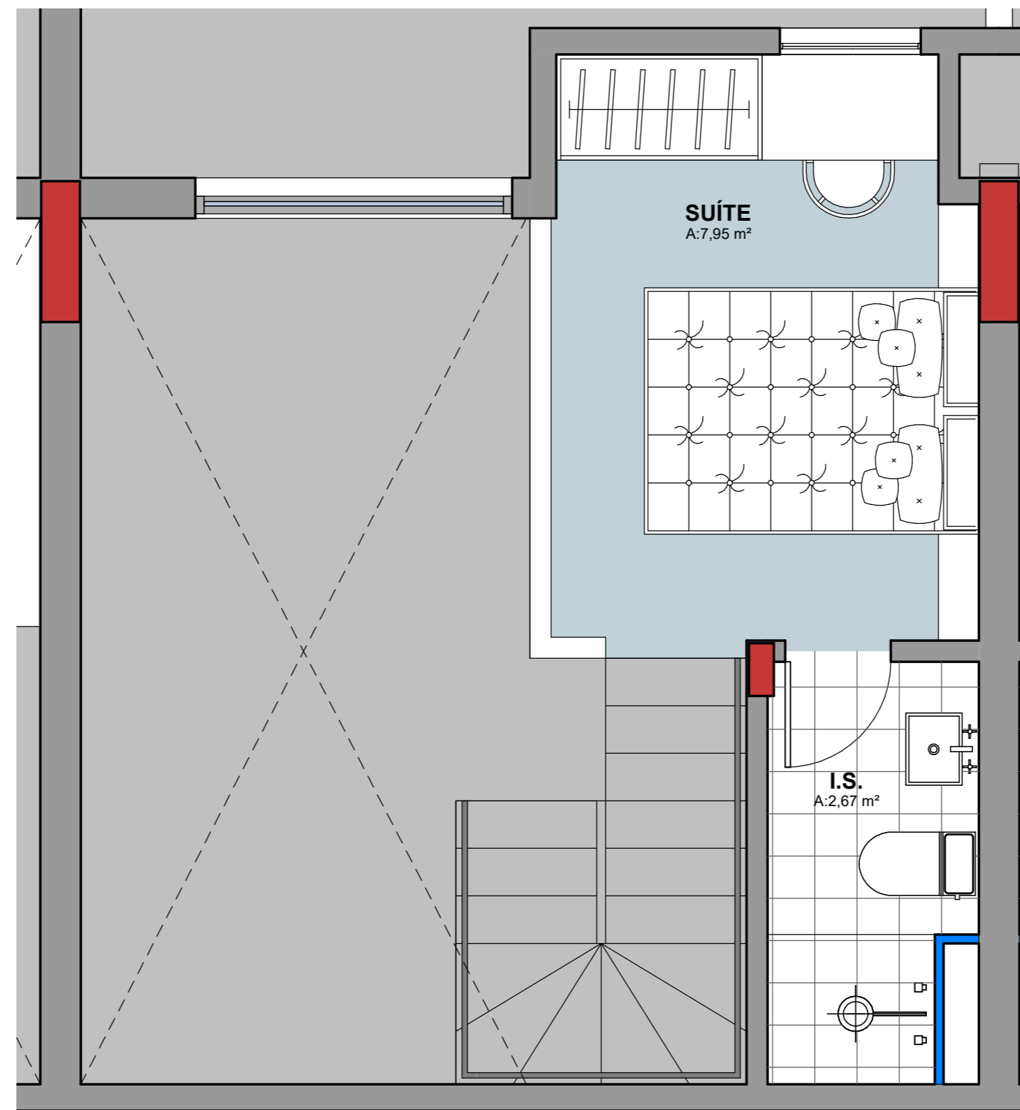
MEZANINO - APTO 107 ESCALA 1 : 30
