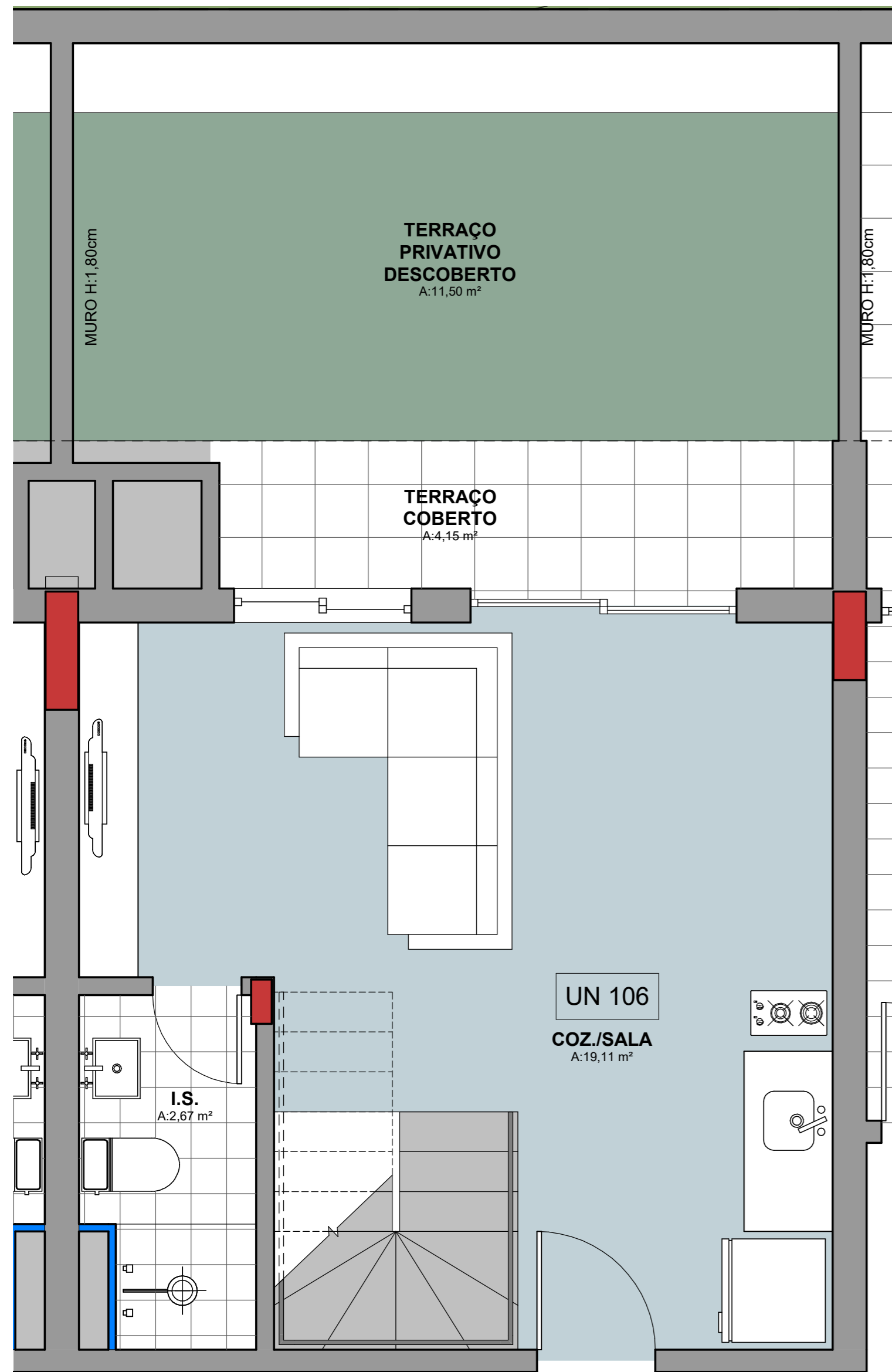
APTO 106 ESCALA 1 : 30
