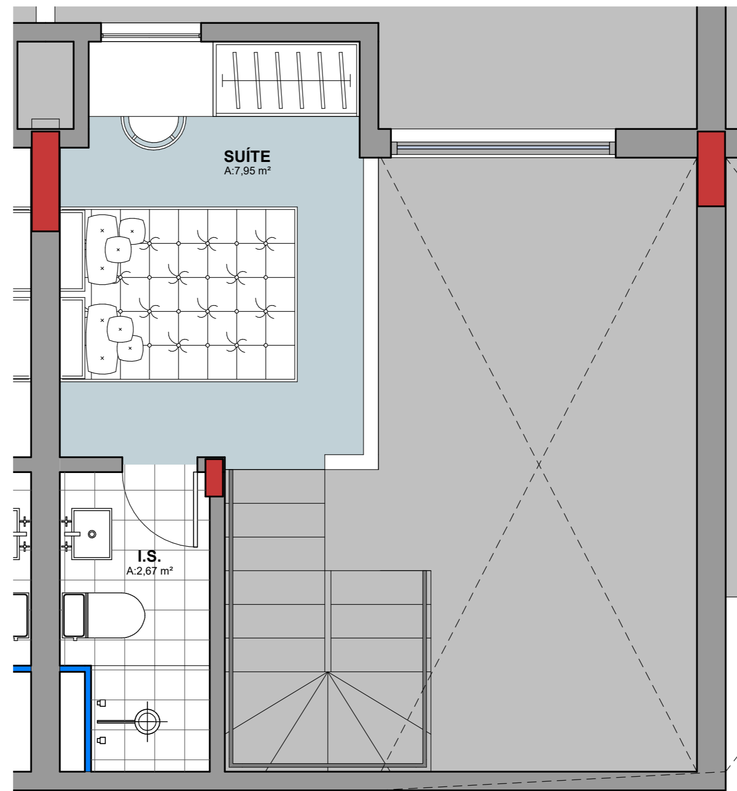
MEZANINO - APTO 106 ESCALA 1 : 30
