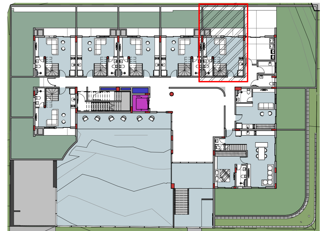
1 - E-01 - TÉRREO - 106 ESCALA 1 : 250
