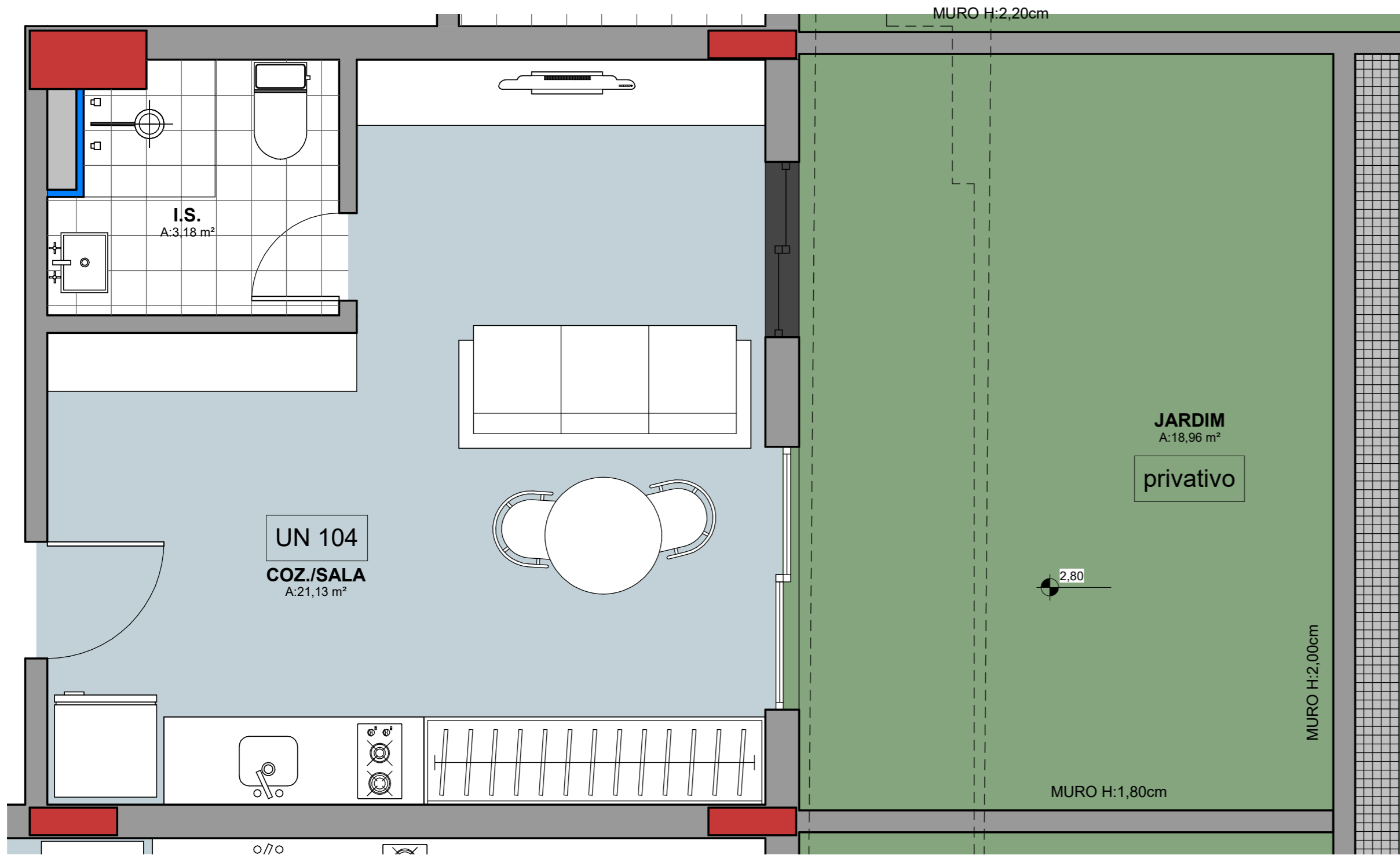
APTO 104 ESCALA 1 : 30
