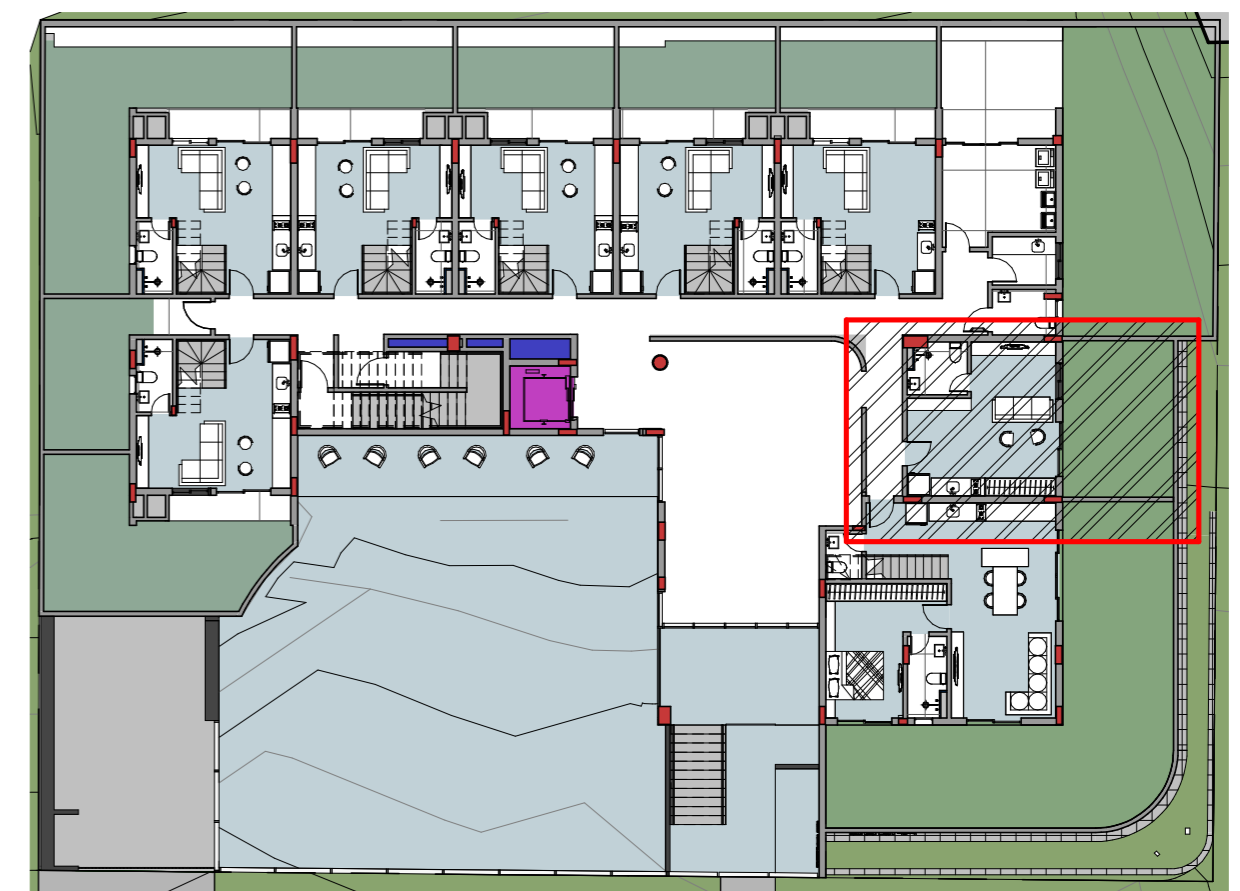
1 - E-01 - TÉRREO - 104 ESCALA 1 : 250
